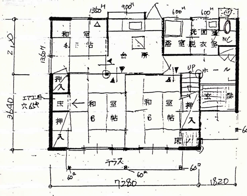
1階平面図
